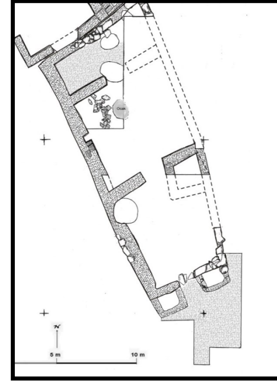
Küllüoba Höyüğü Megaron yapısı planı (M.Ö. 3. Binyıl)
